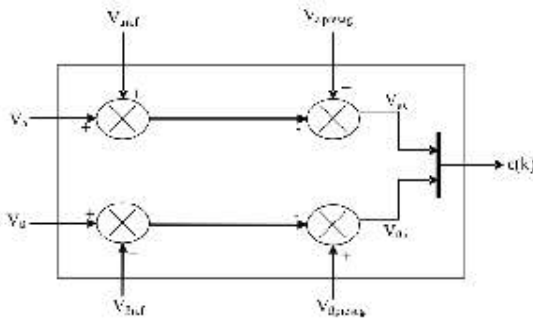
Fig. 8. Error generator
